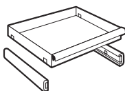
Ripiano scorrevole Mod. 110-300: 37x455x376 Mod. 350: 37x530x400 Mod. 450: 20x550x430
